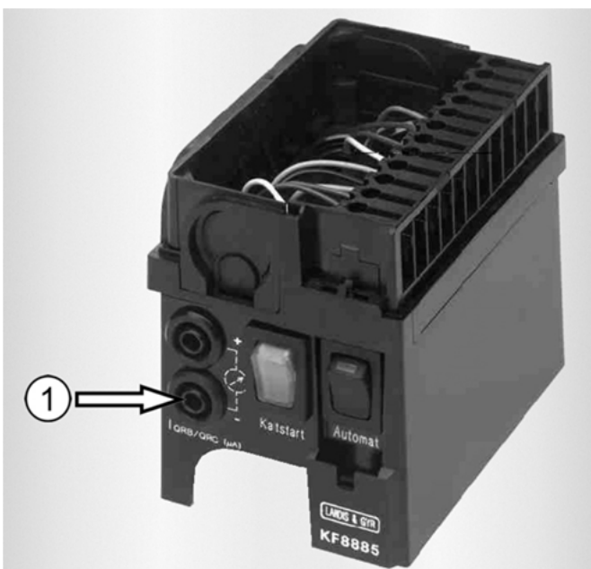
Abb. 41: Prüfsockel KF 8885 (Sach-Nr. 95.95215-0085) Messanschluss Lichtfühler ①
