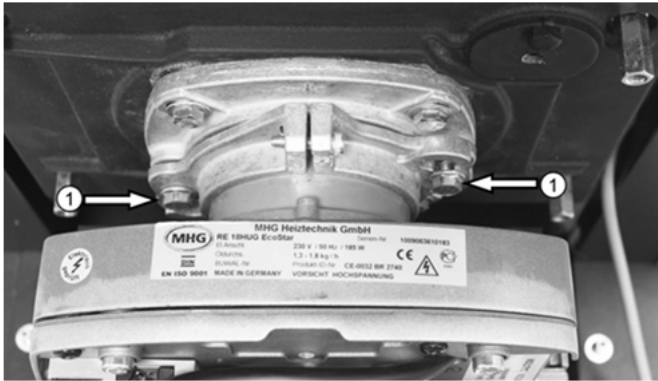
Abb. 31: Brennerbefestigungsschrauben
