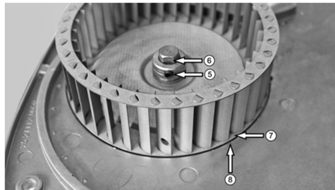
Abb. 40: Axiale Positionierung des Gebläserades
