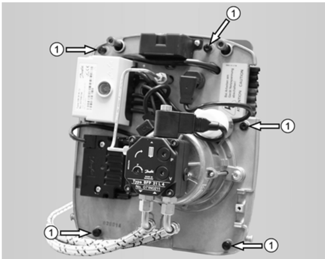
Abb. 32: Gehäusedeckel mit 5 Schnellverschluss-Schrauben ①
