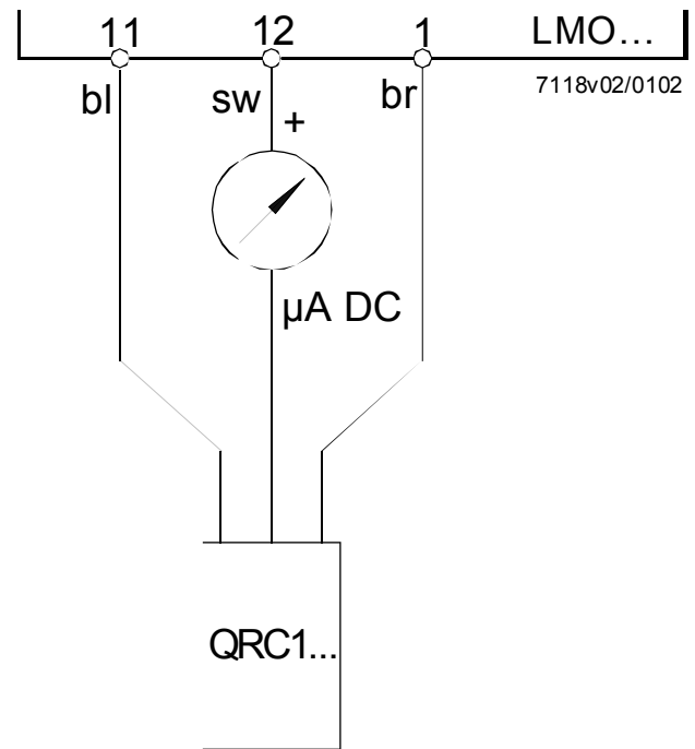
Abb. 42: Mess-Schaltung zur Fühlerstrommessung
