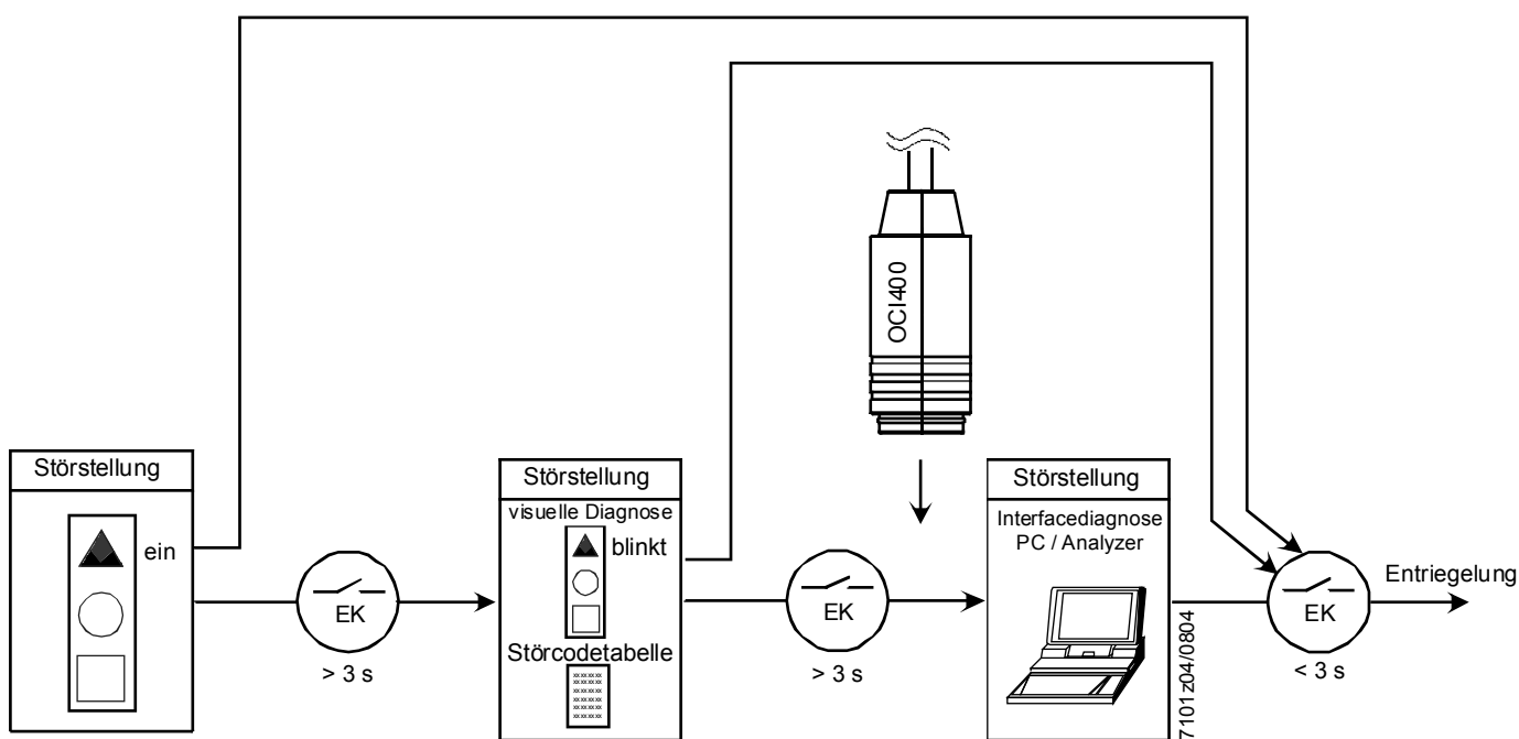
Abb. 44: Ablauf Störursachendiagnose EK = Entstörtaster
