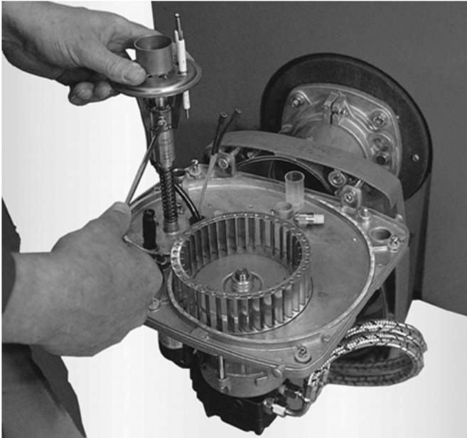
Abb. 34: Demontage Mischsystem
