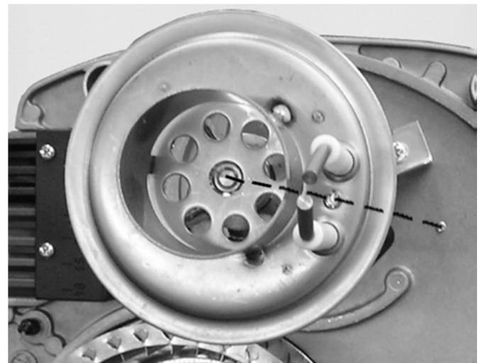
Abb. 37: Mischsystempositionierung und Ausrichtung Zündelektrode
