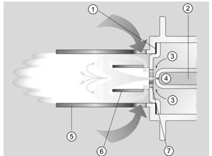
Abb. 48: Verbrennungsablauf Raketenbrenne®
