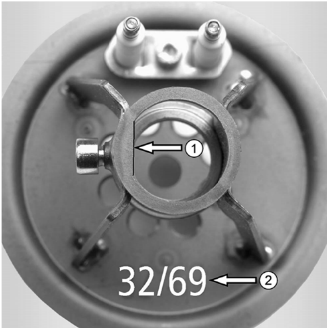
Abb. 35: Rückansicht Mischsystem mit Verdrehsicherung ① und Mischsystemgröße ②
