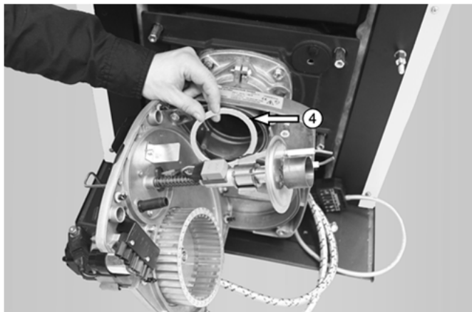
Abb. 39: Einsetzen eines Dichtringes (4) ins Stützrohr
